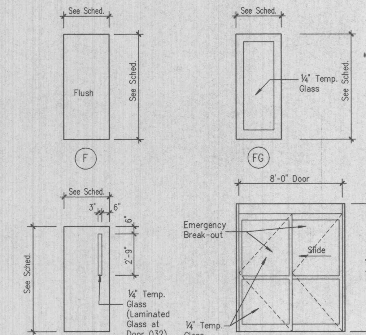
14 DOOR TYPES
