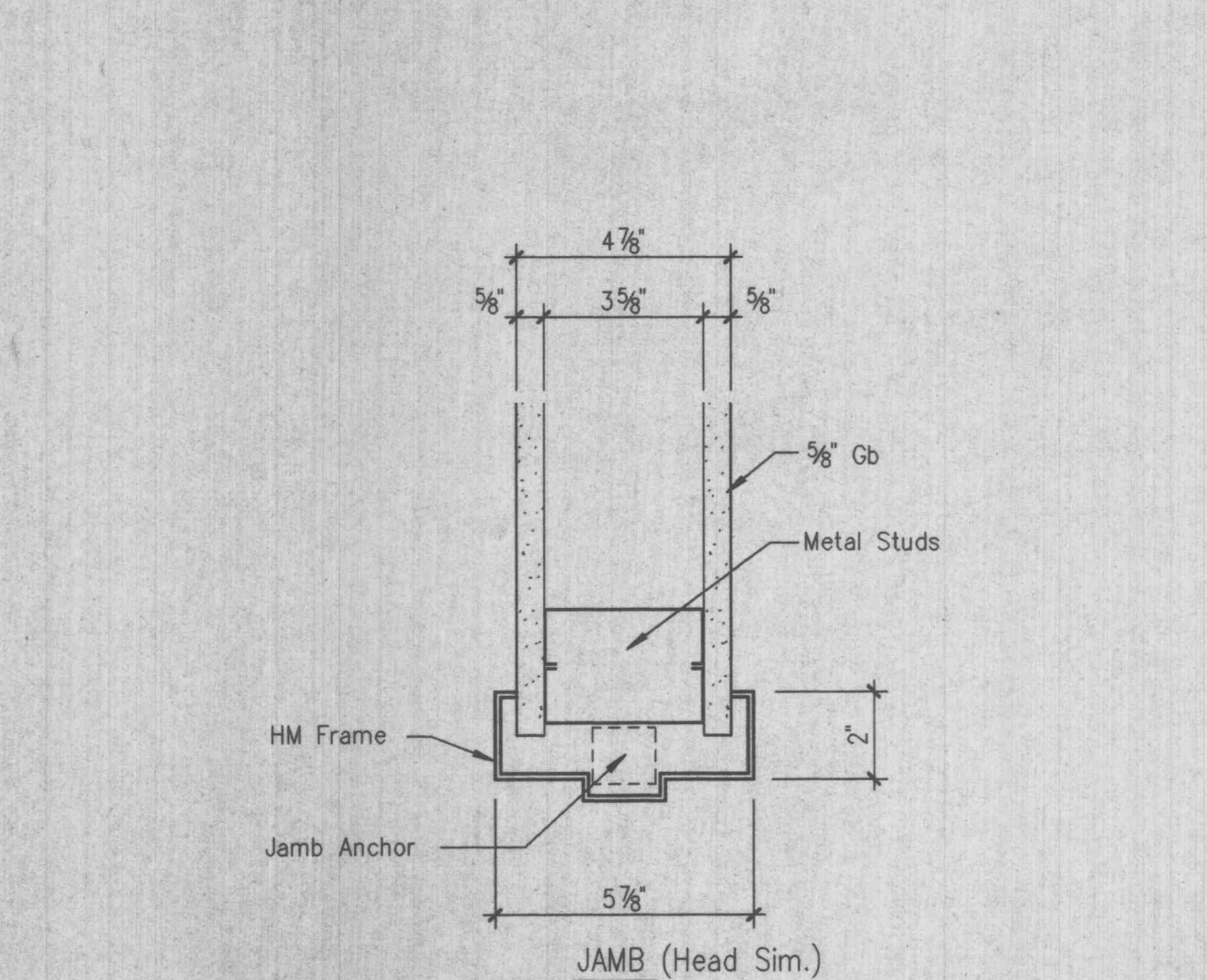
11 HM DOOR FRAME
