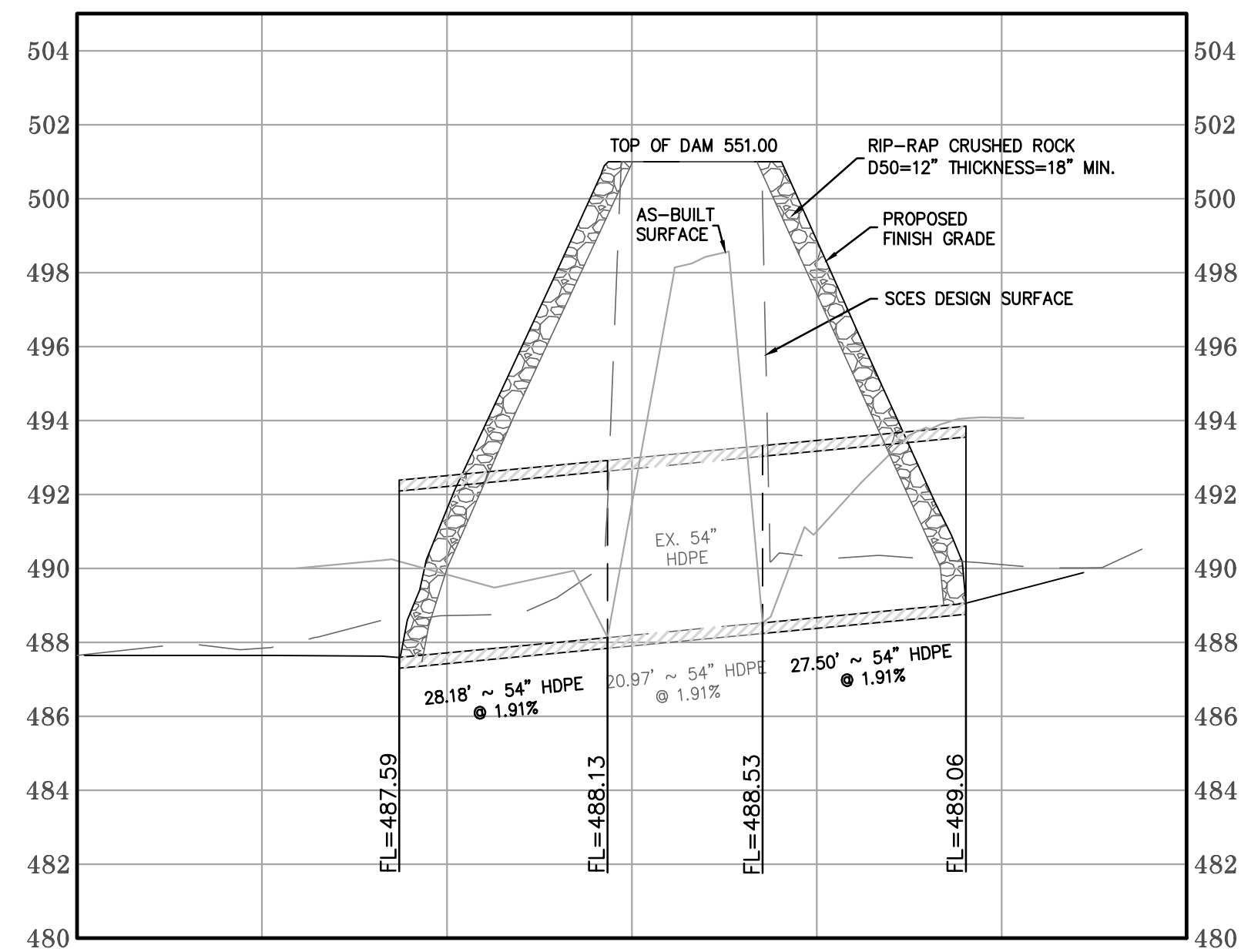
EOP 501-502 E - CROSS SECTION N.T.S.
