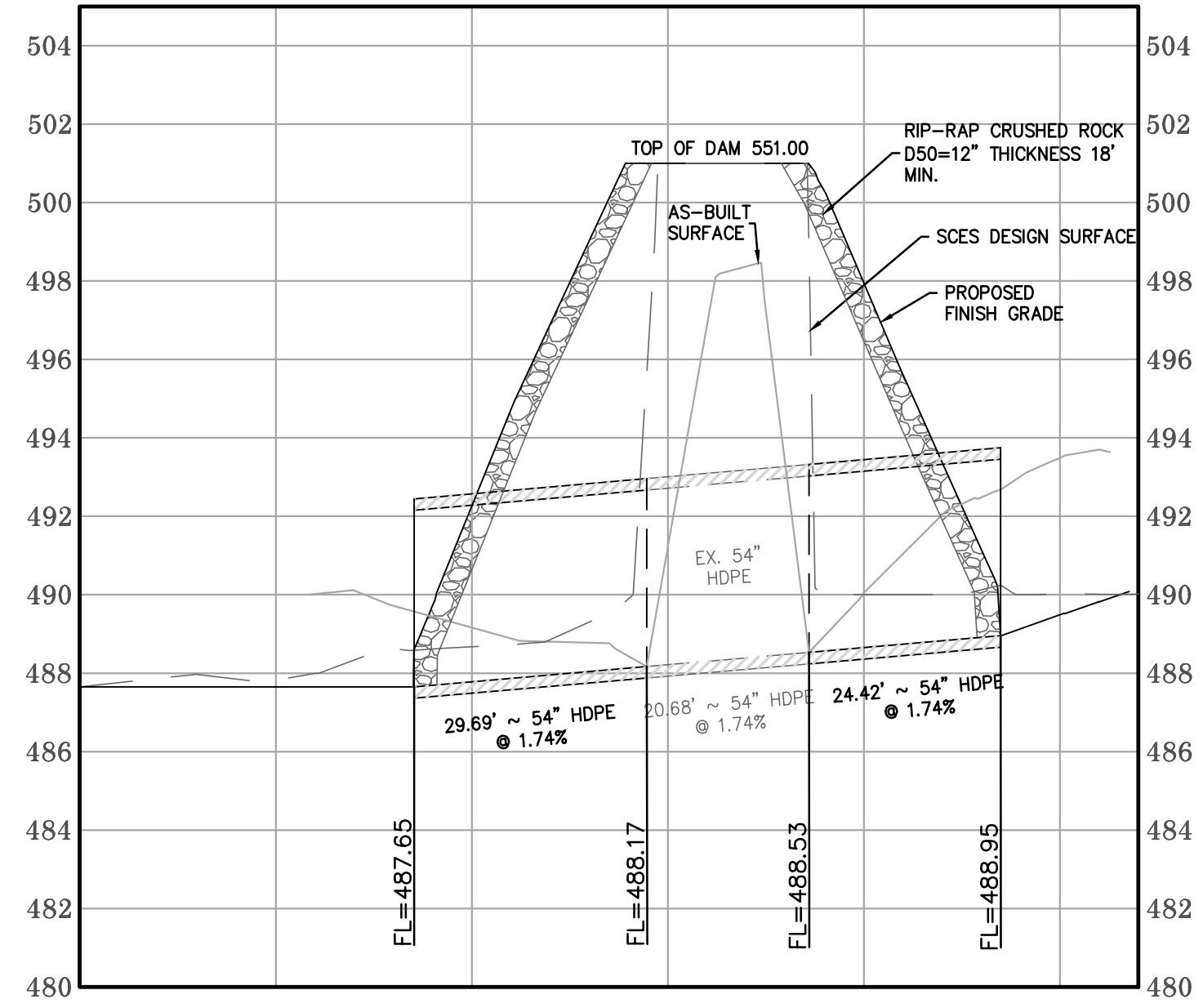
EOP 501-502 W - CROSS SECTION N.T.S.
