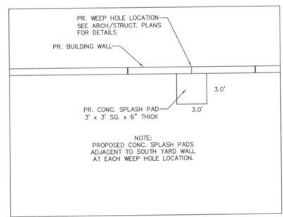
SPLASH PAD DETAIL SCALE: 1" = 5'
