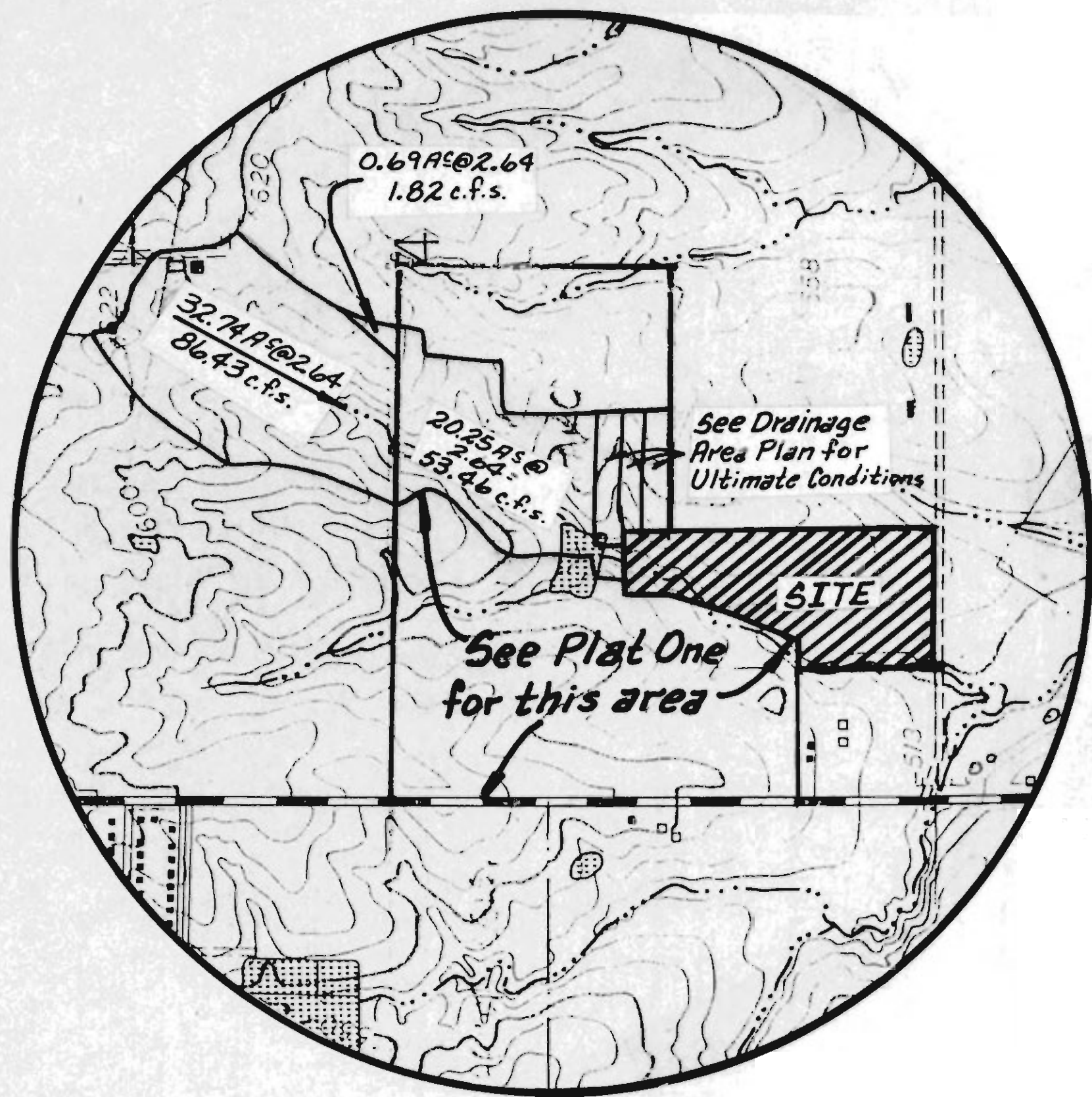
OFF-SITE DRAINAGE AREA MAP N.T.S.
