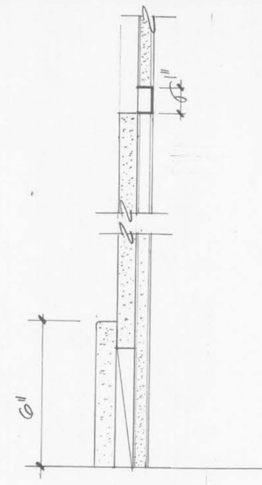
1 P.C. T2 BASE 3" x 1'-0"
