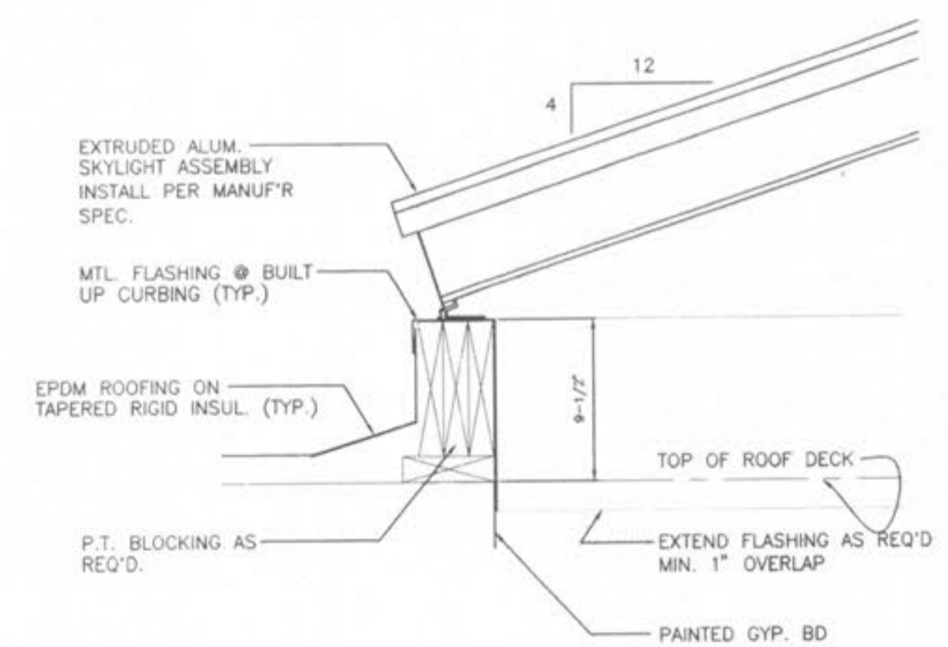
DETAIL • SKYLIGHT (TYP.) NTS
