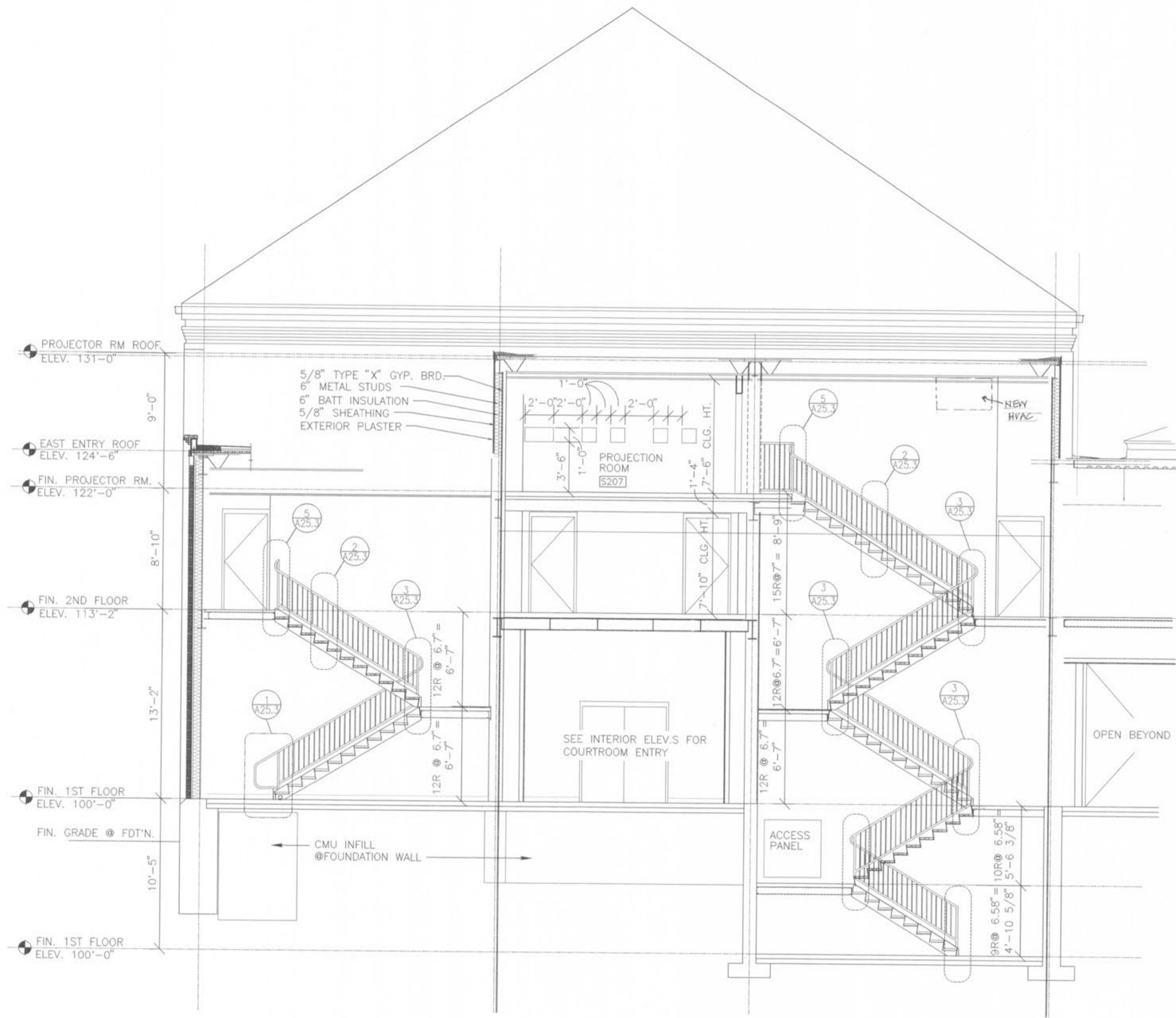
4 SECTION • STAIRS E + F SCALE: 1/4" = 1'-0"
