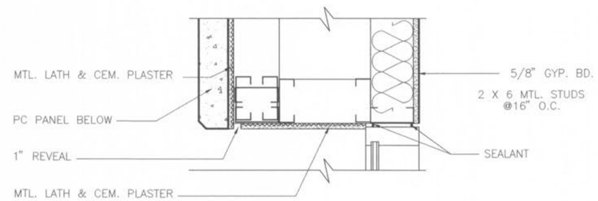
4 PLASTER JAMB A-39.1 SCALE: 1 1/2"=1'-0"
