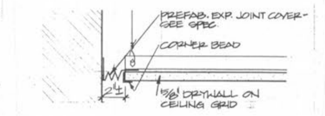
10 EXP. JT. @ DRYWALL CLG./WALL SCALE 3/4"=1'-0"
