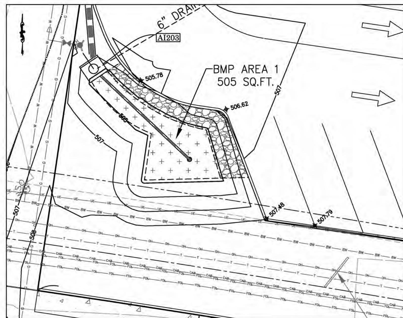
BMP AREA 1 SCALE: 1"=10'
