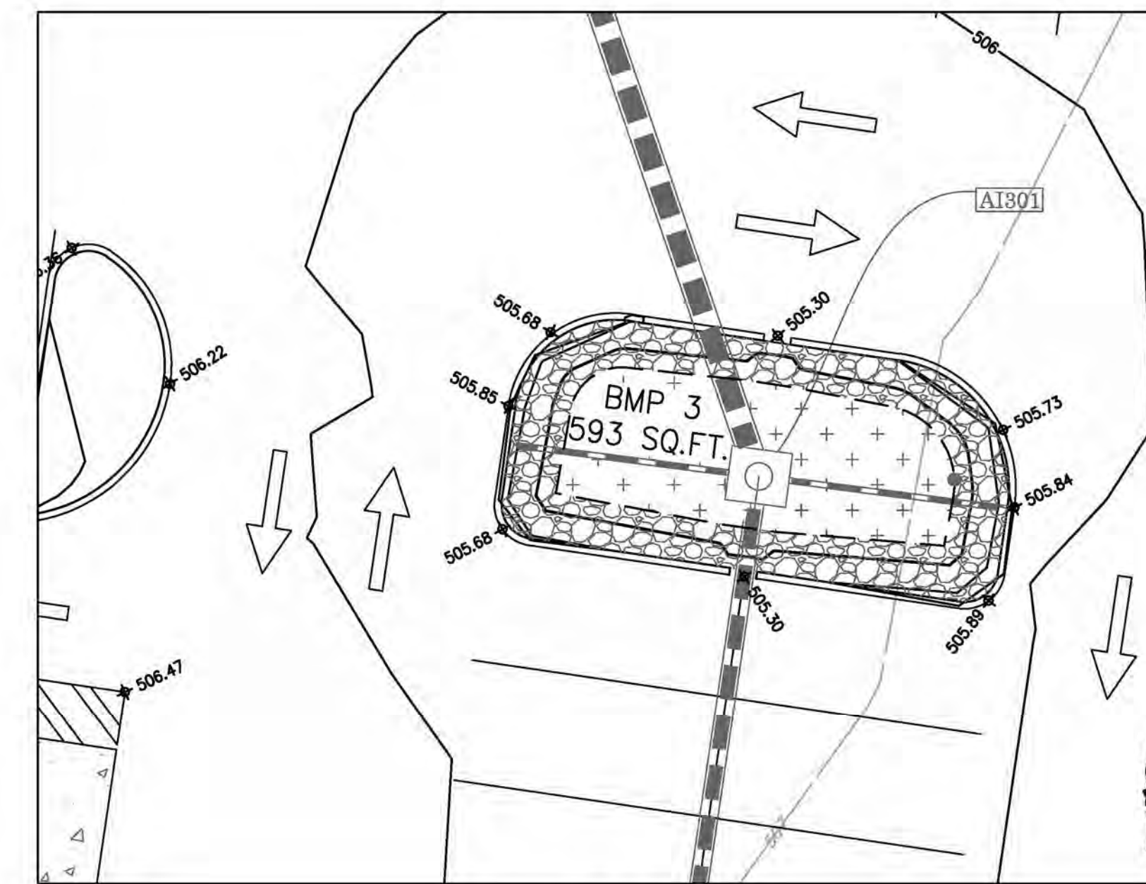
BMP AREA 3 SCALE: 1"=10'
