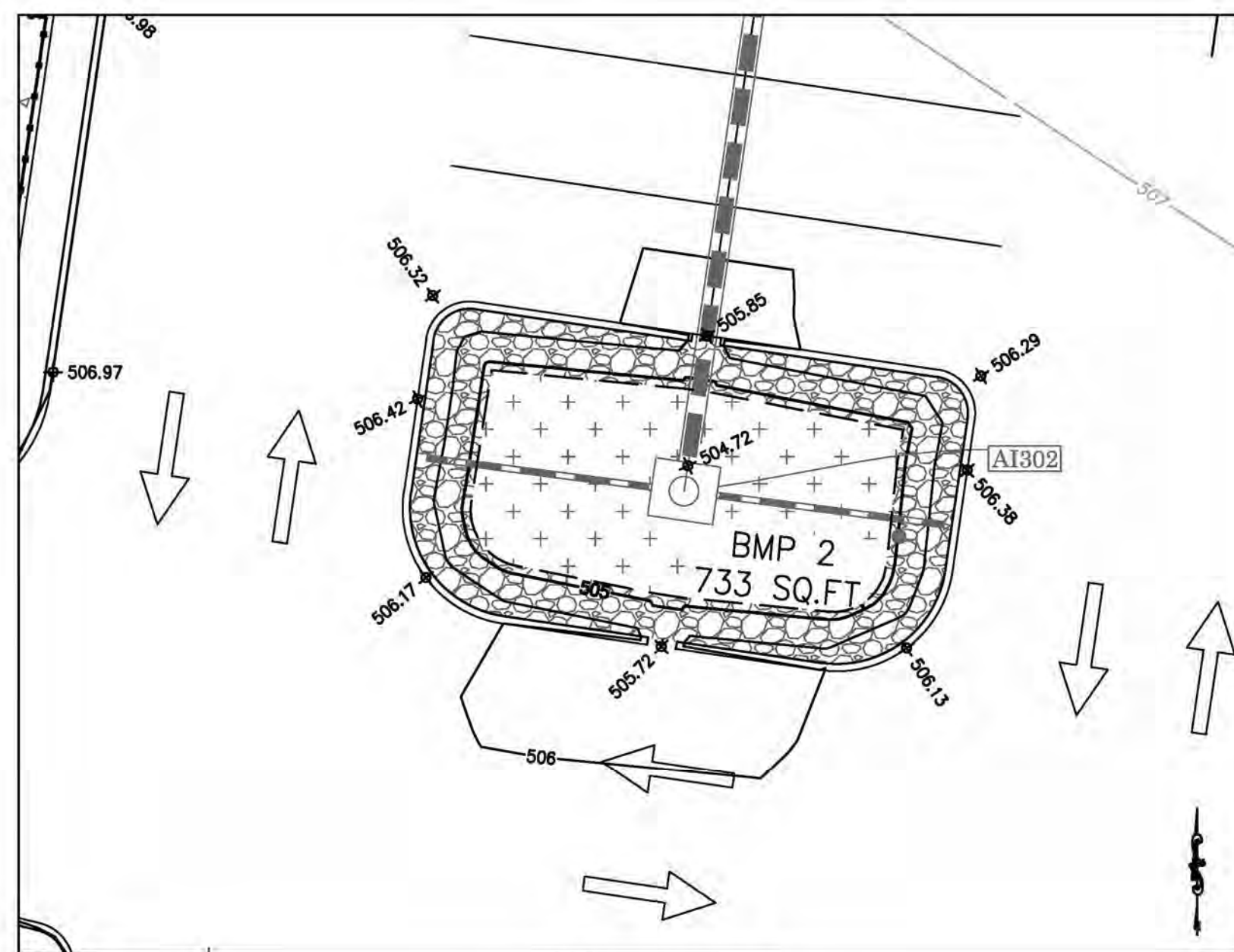
BMP AREA 2 SCALE: 1"=10'
