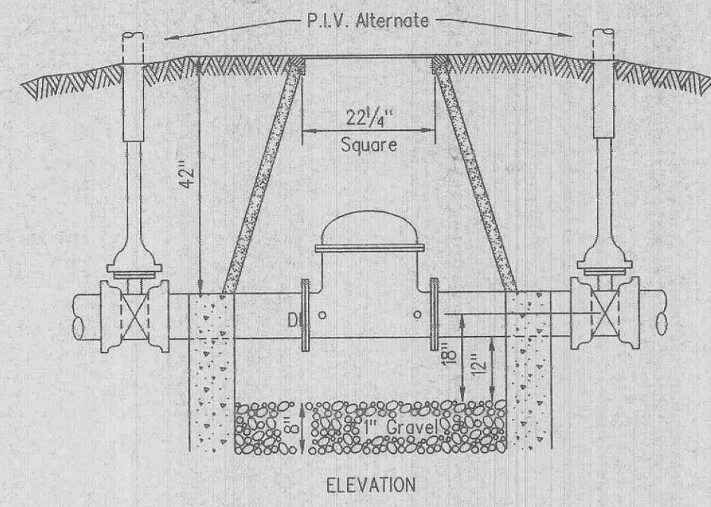
ELEVATION
