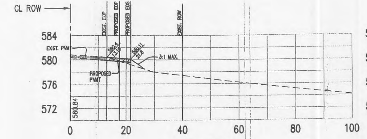
STA: 495+00
