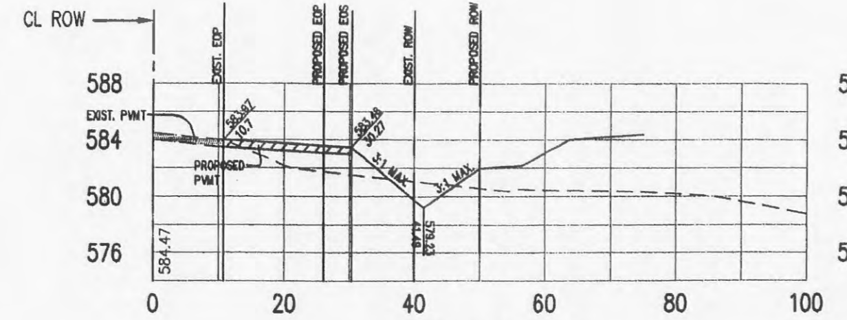
STA: 491+00
