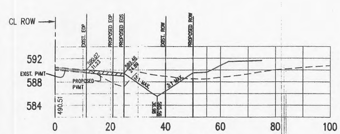
STA: 487+00
