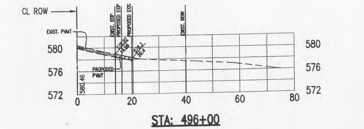
STA: 496+00
