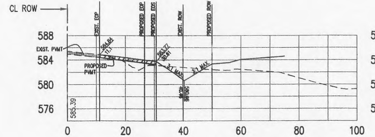
STA: 490+50
