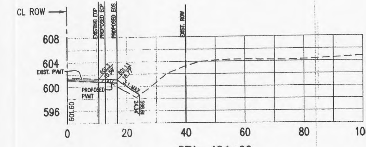
STA: 484+00
