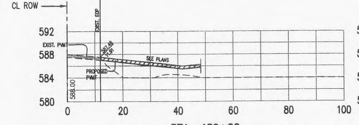
STA: 489+00
