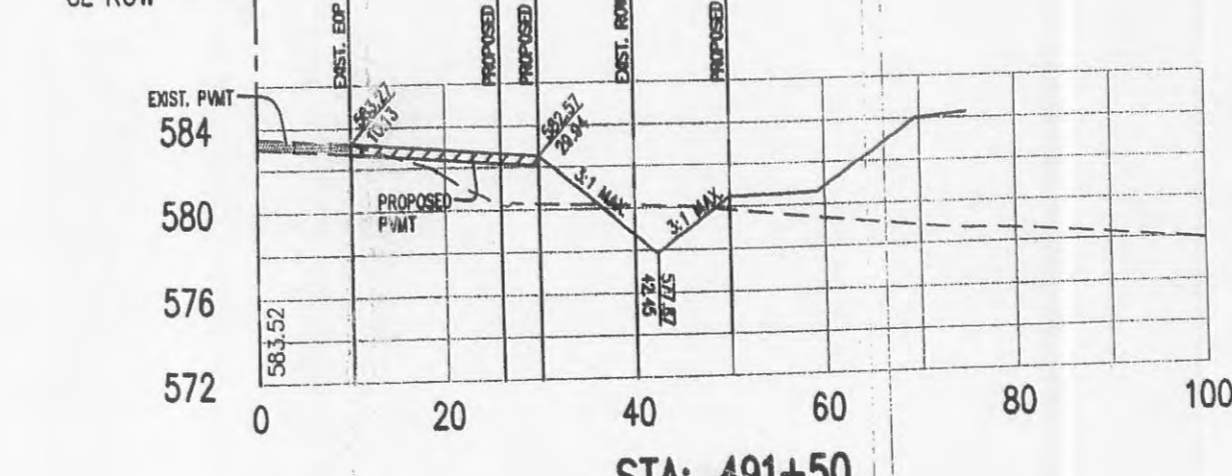
STA: 491+50
