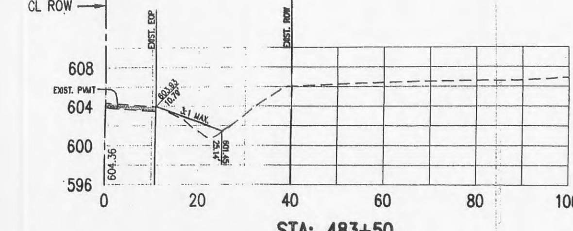
STA: 483+50
