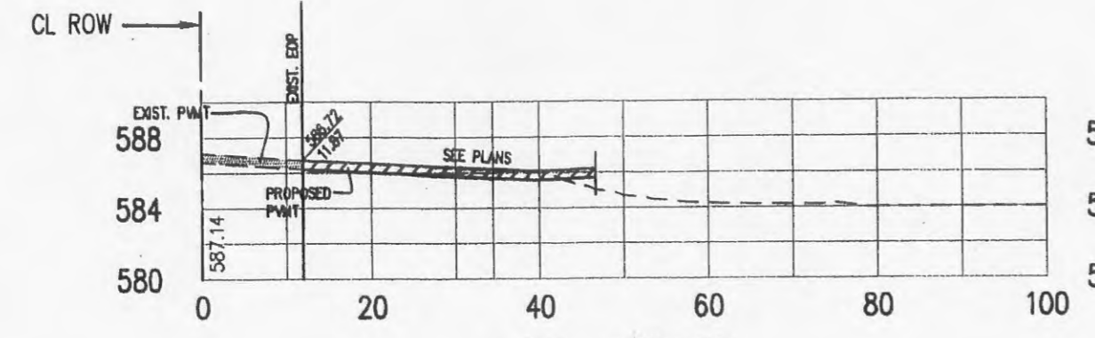
STA: 489+50
