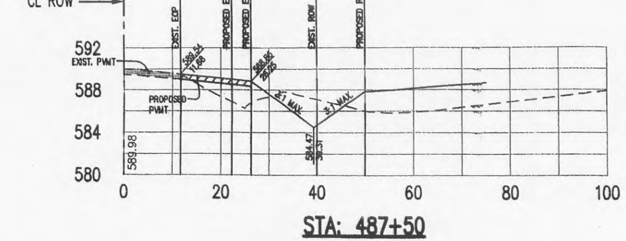
STA: 487+50
