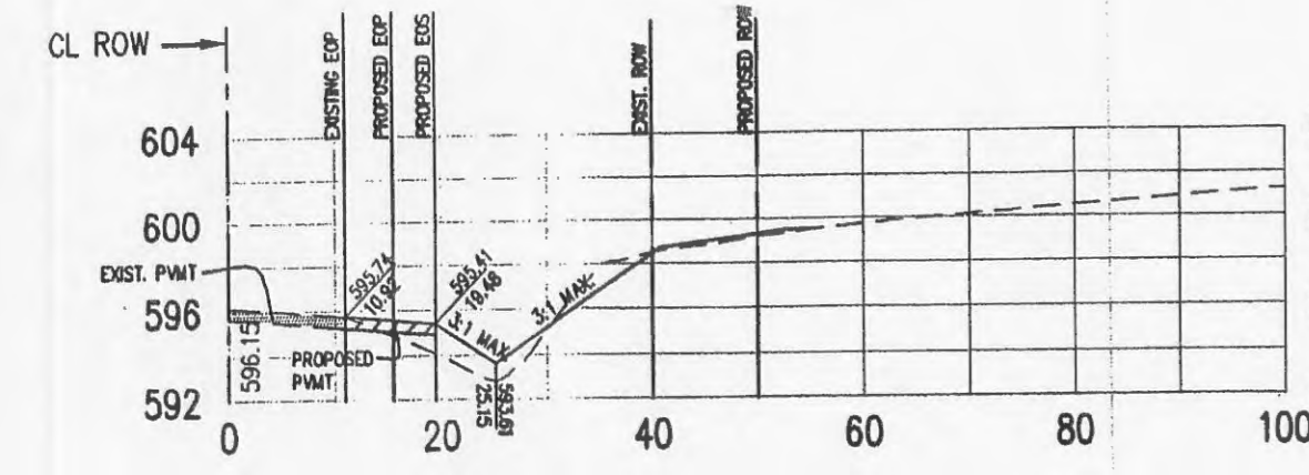
STA: 485+00
