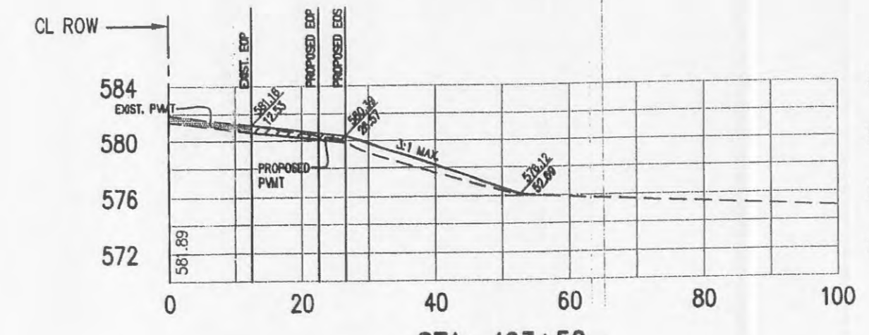
STA: 493+50
