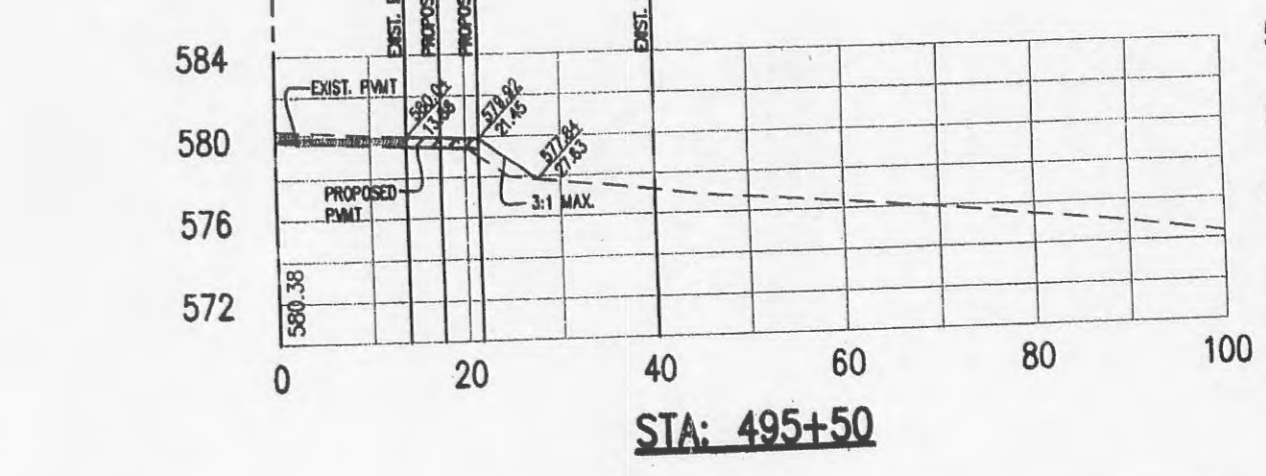
STA: 495+50
