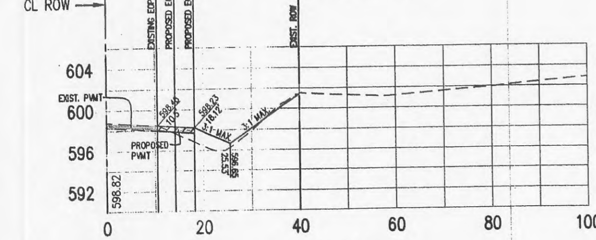
STA: 484+50
