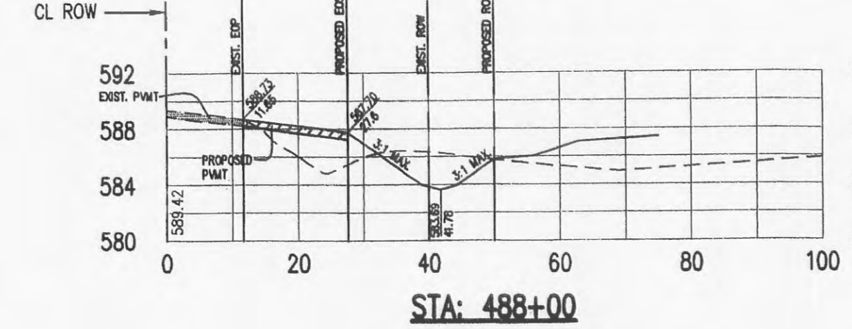
STA: 488+00
