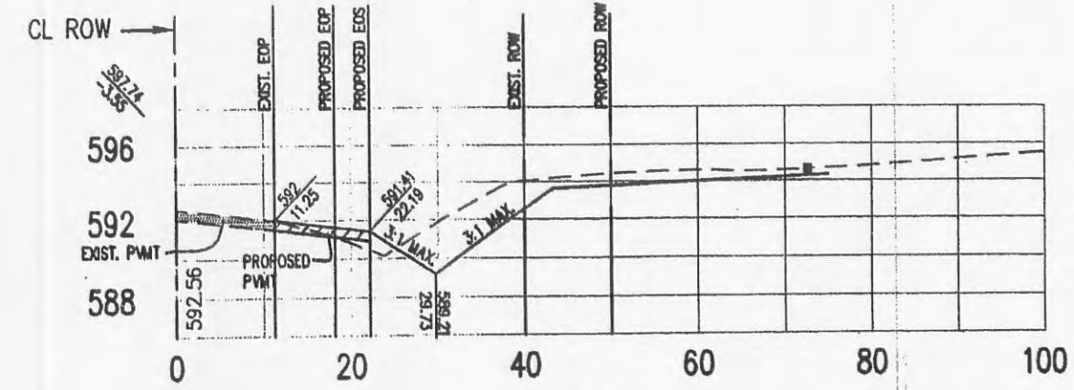
STA: 486+00
