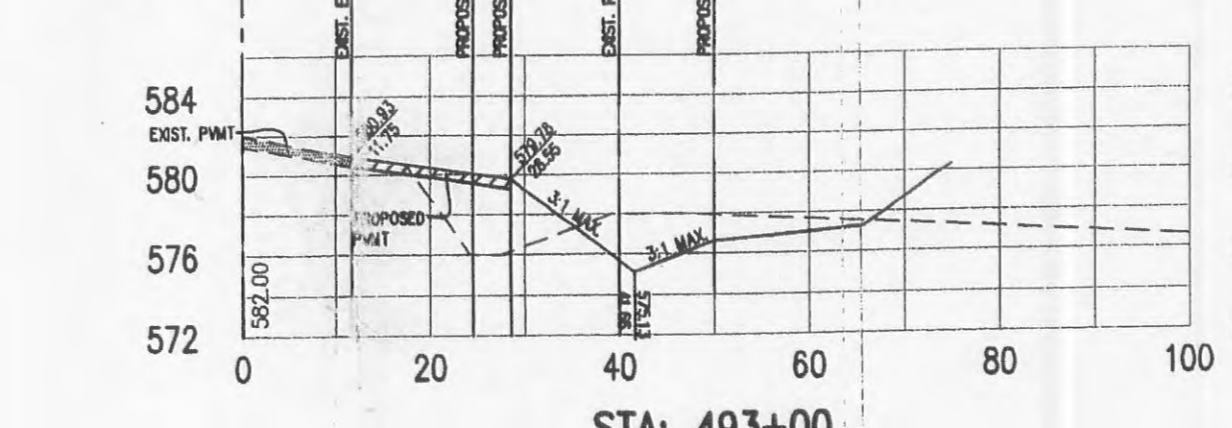
STA: 493+00
