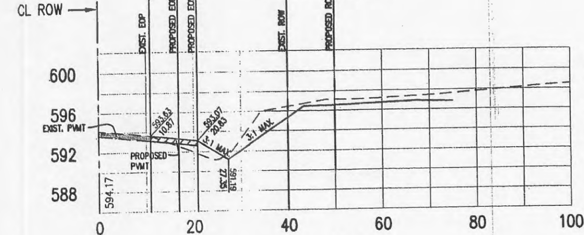
STA: 485+50
