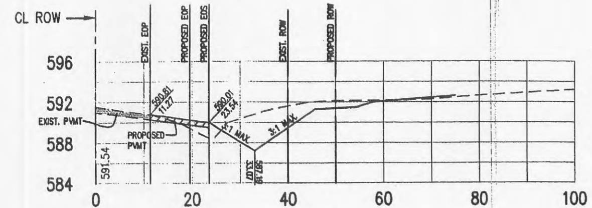
STA: 486+50
