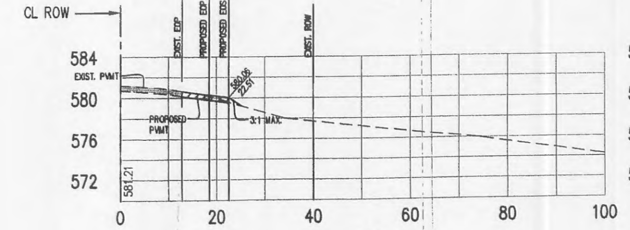
STA: 494+50
