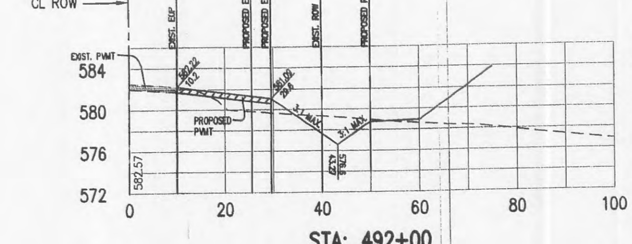
STA: 492+00
