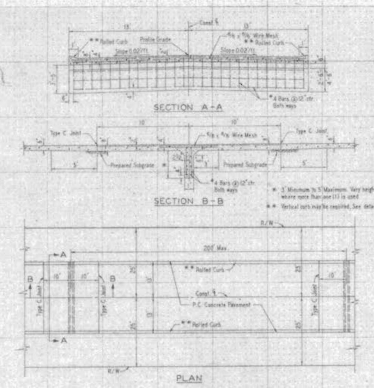
PAVEMENT LUG DETAIL
