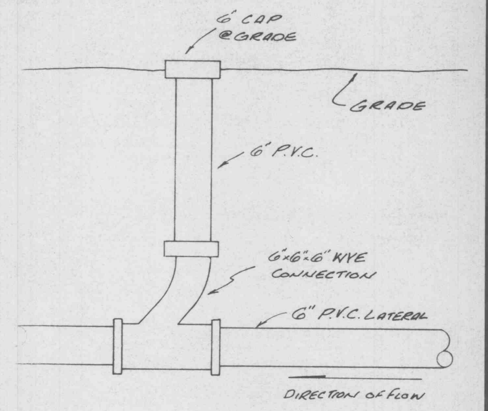
CLEAN-OUT DETAIL N.T.S.
