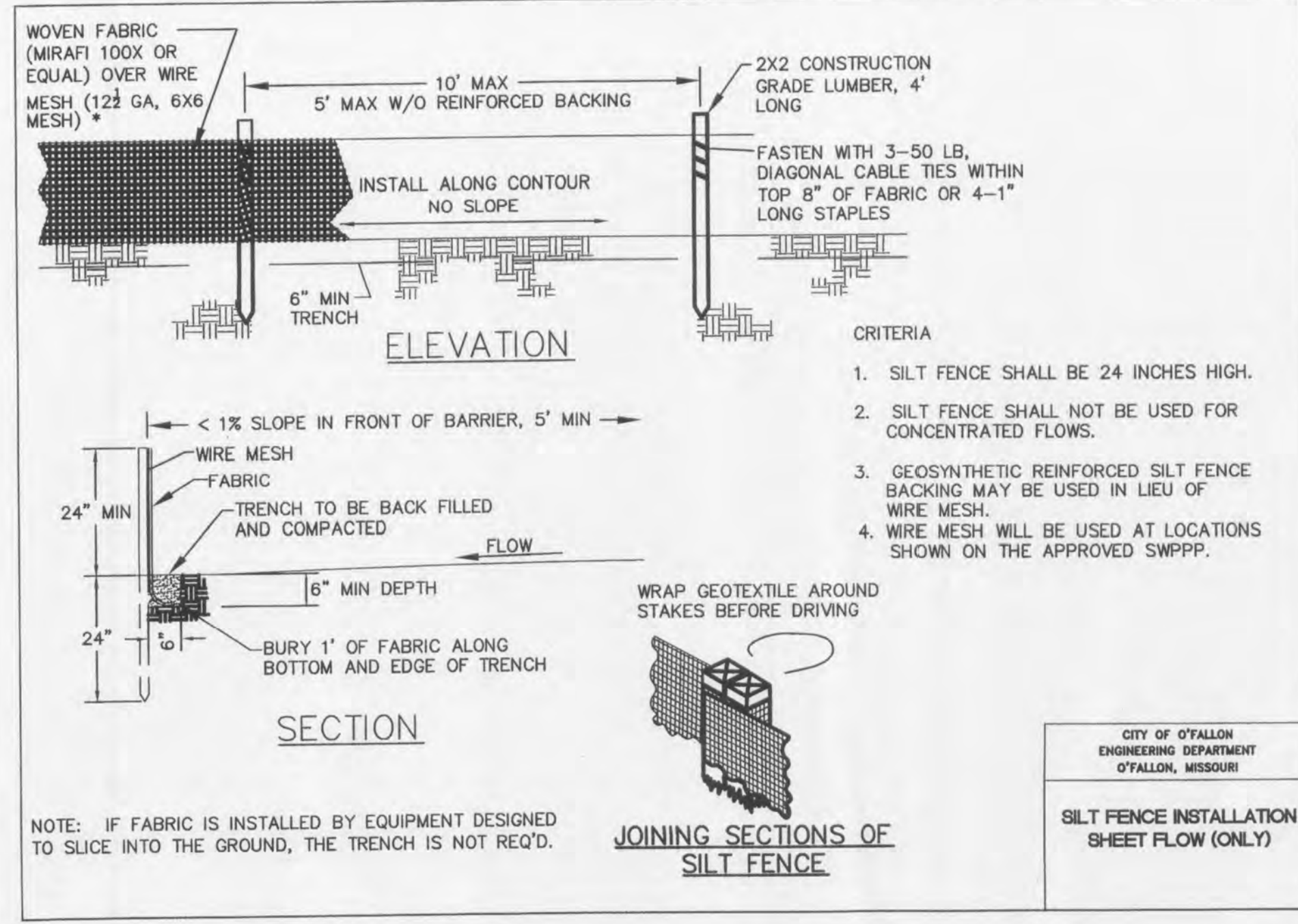
3 SILT FENCE C502 N.T.S.
