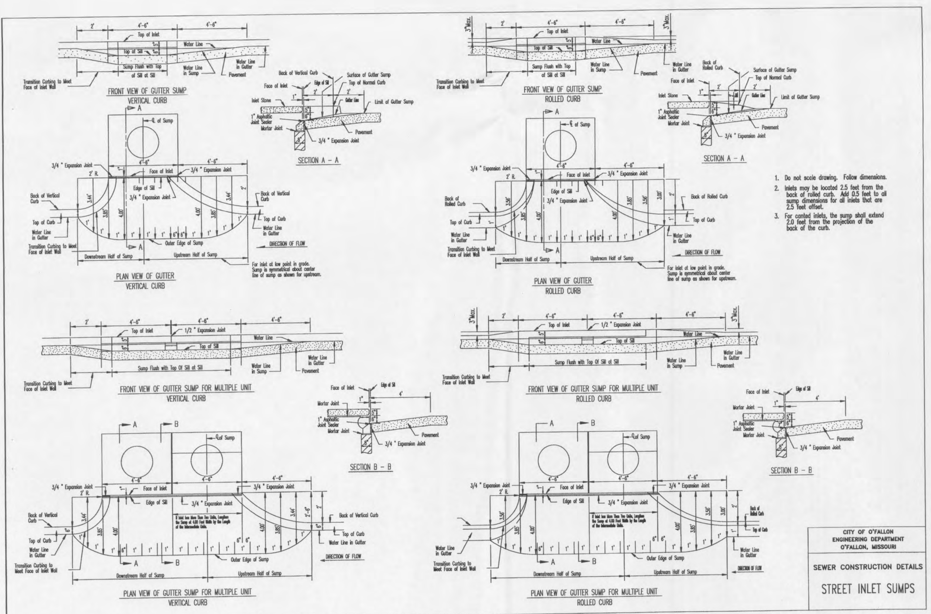
2 STREET INLET SUMPS C502 N.T.S.
