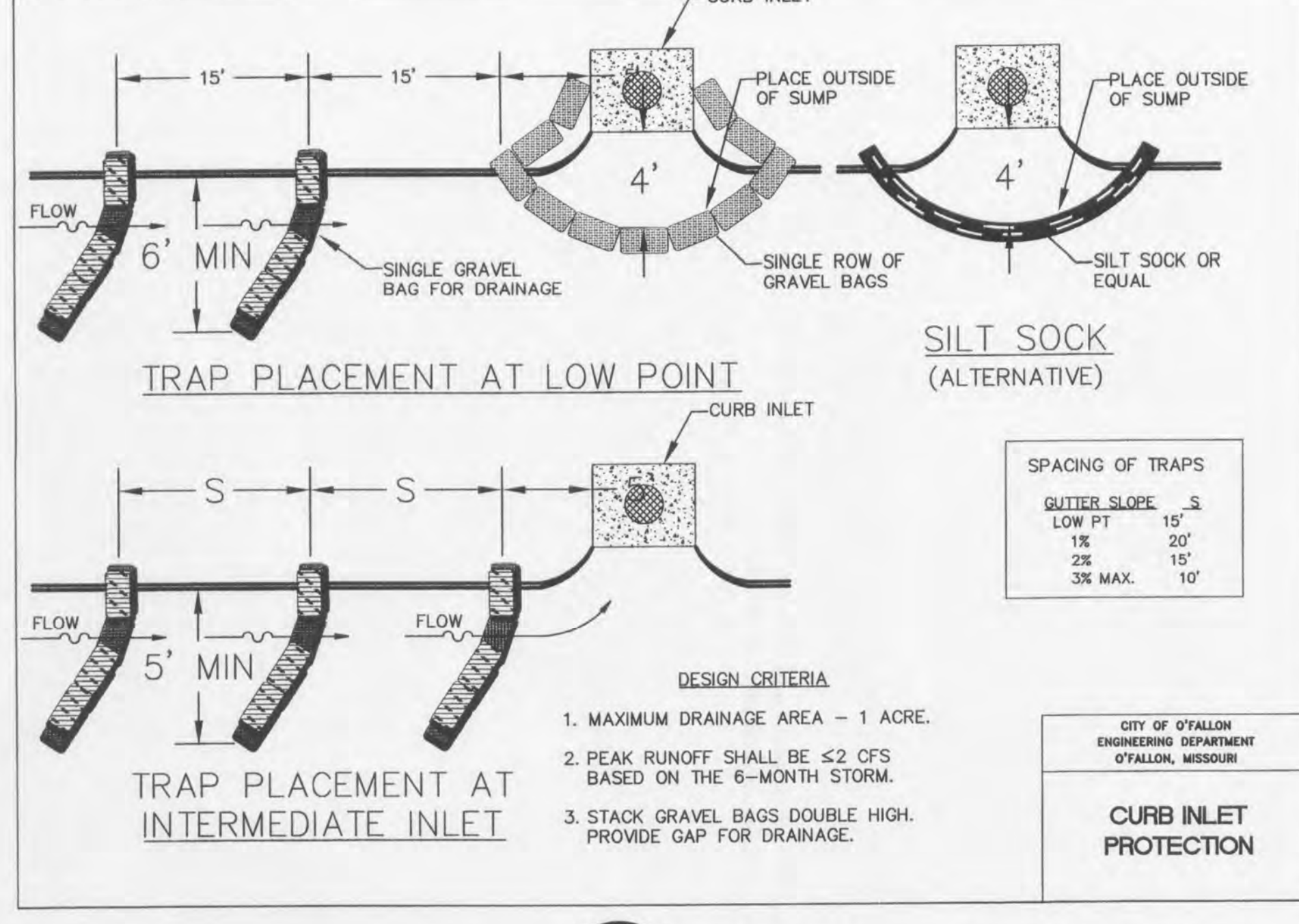
5 CURB INLET PROTECTION C502 N.T.S.
