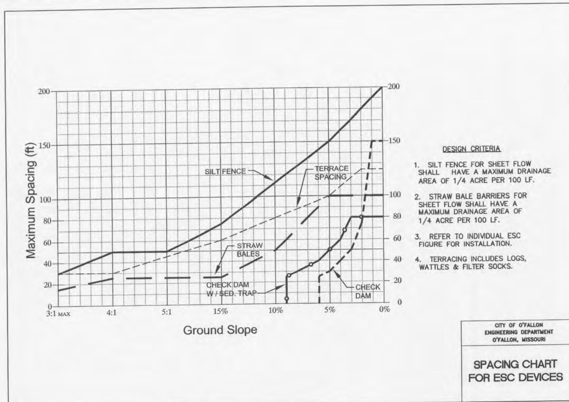
1 SPACING CHART C502 N.T.S.
