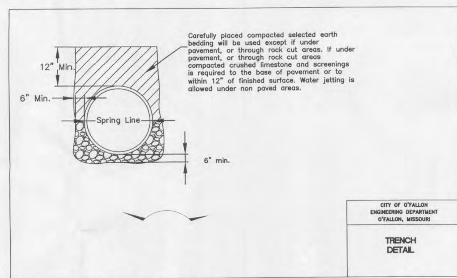
4 TRENCH DETAIL C502 N.T.S.
