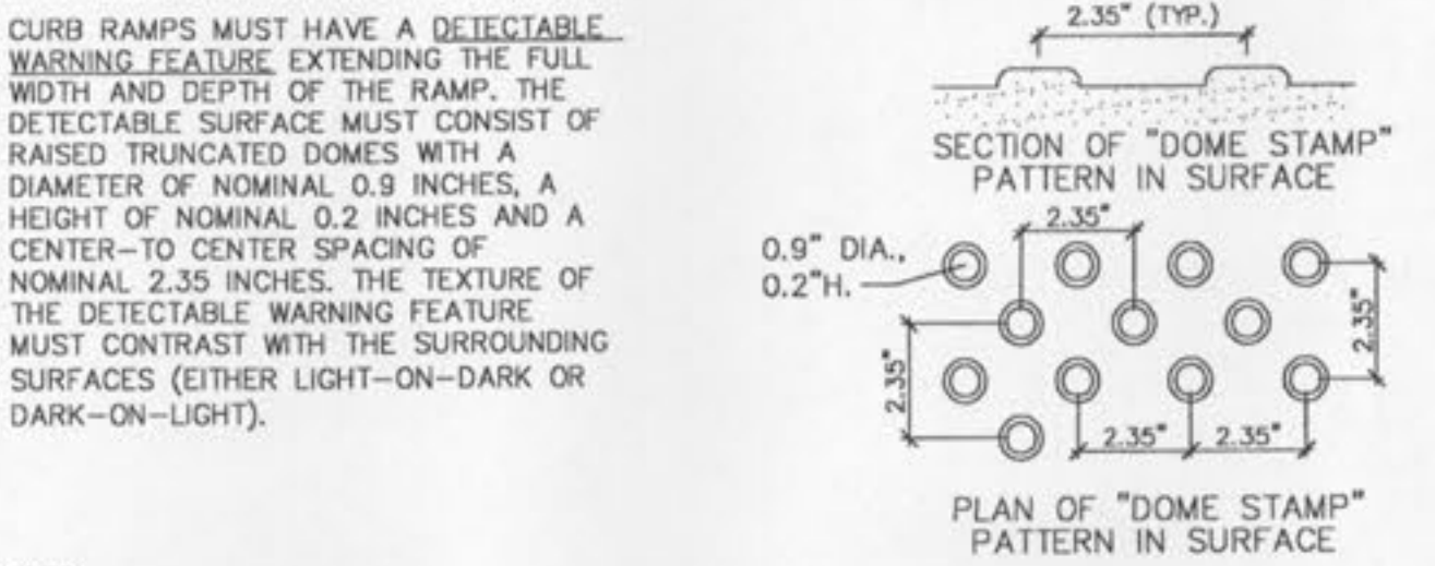
7 DETECTABLE WARNING SURFACE DETAIL SCALE: N.T.S. REF. DWG. C3.0
