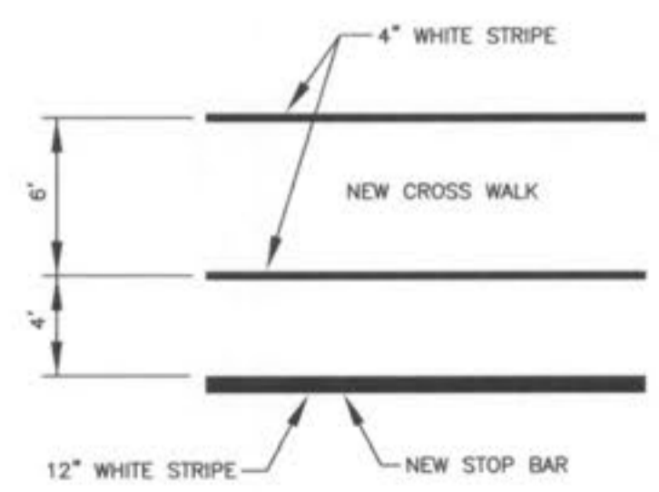
CROSS WALK DETAIL N.T.S.
