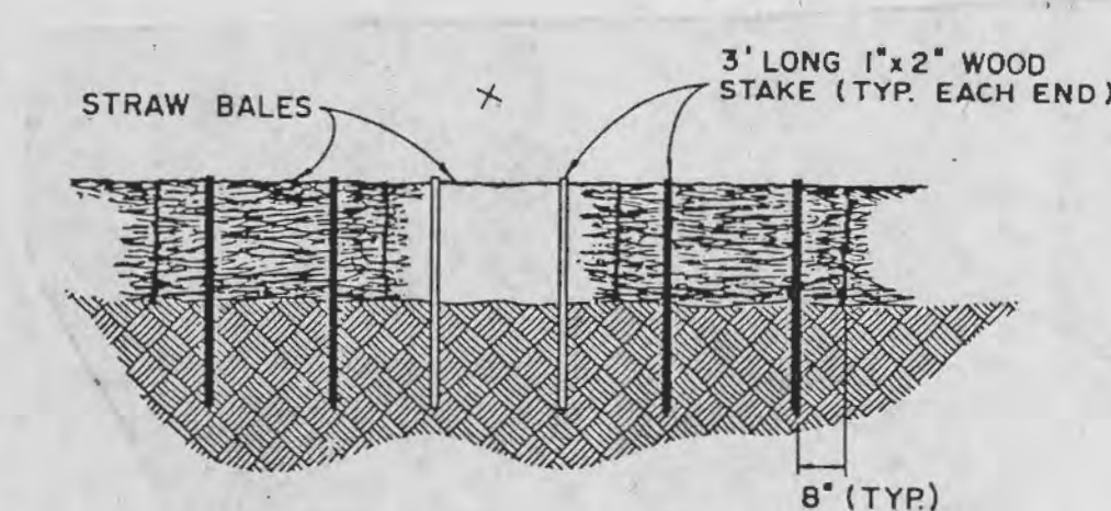
STAKED BALE DETAIL N.T.S.
