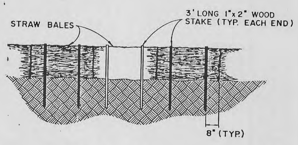
STRAKED BALE DETAIL N.T.S.
