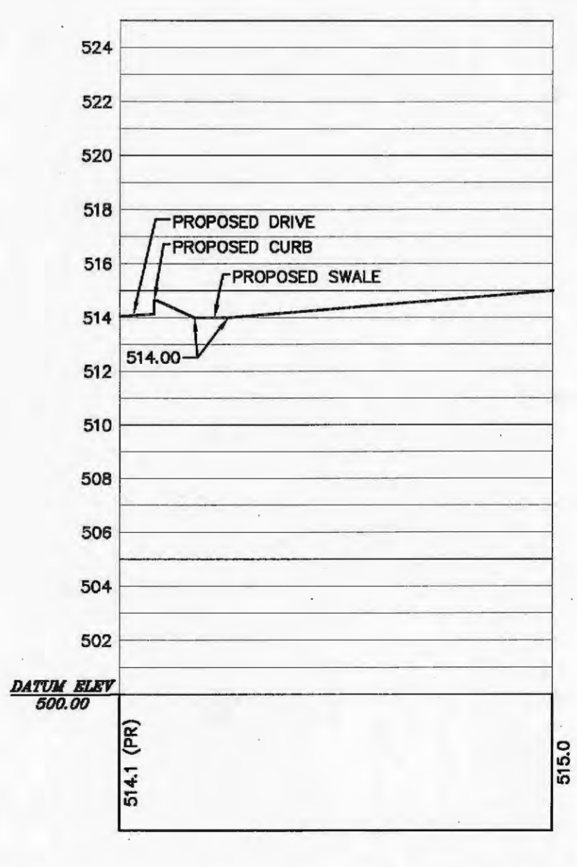
STORM SWALE CROSS SECTION HOR.: 1"=20' VERT.: 1"=5'
