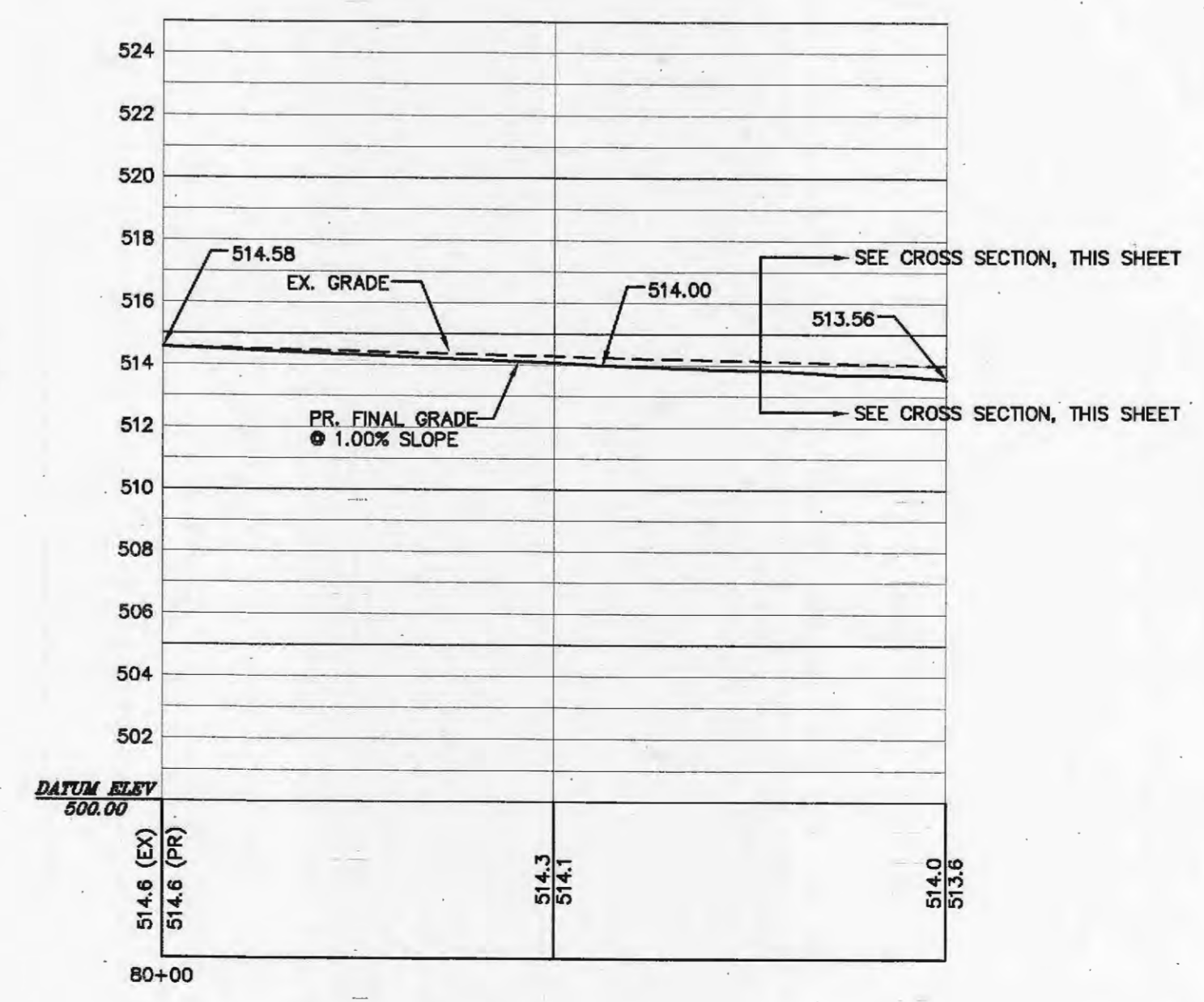
STORM SWALE PROFILE HOR.: 1"=20' VERT.: 1"=5'
