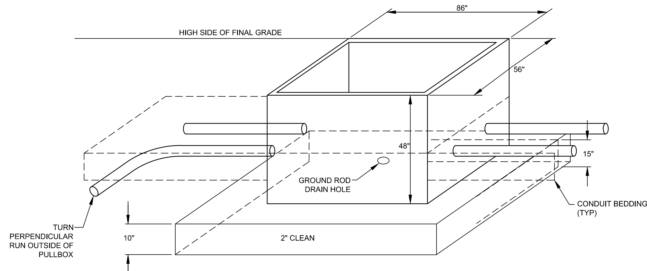
PULLBOX DETAIL SCALE: N.T.S.
