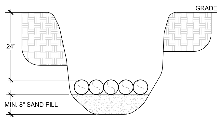
CONDUIT BURIAL DETAIL SCALE: N.T.S.
