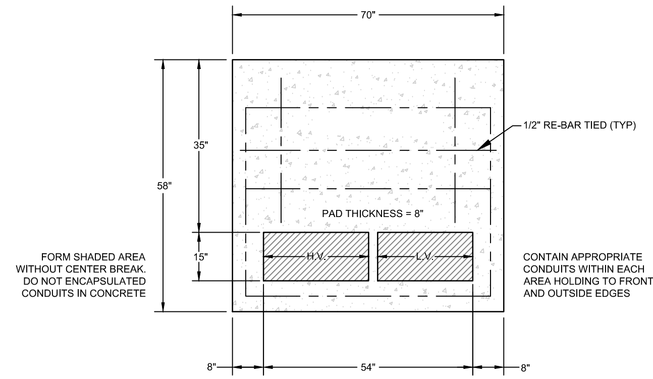
45-75 KVA TRANSFORMER PAD DETAIL SCALE: N.T.S.
