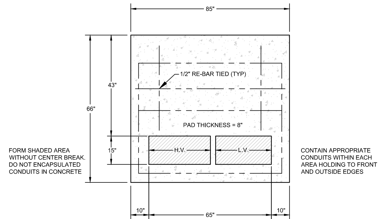
100-500 KVA TRANSFORMER PAD DETAIL SCALE: N.T.S.
