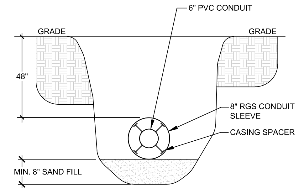
PRIMARY CONDUIT W / SLEEVE BURIAL DETAIL SCALE: N.T.S.
