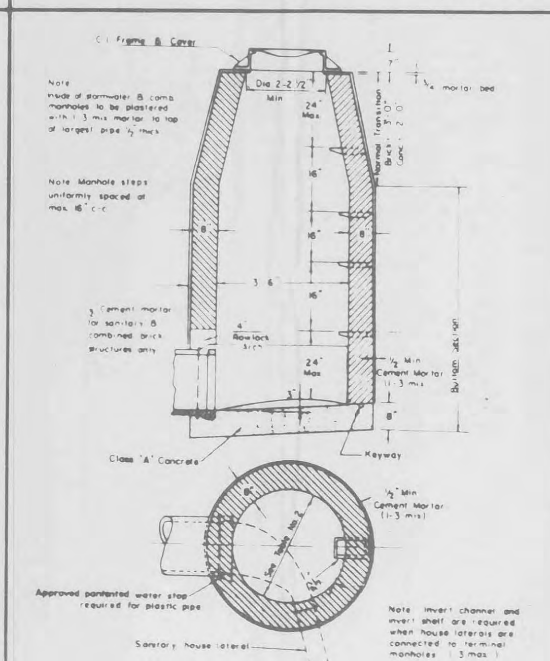
TERMINAL MANHOLE
