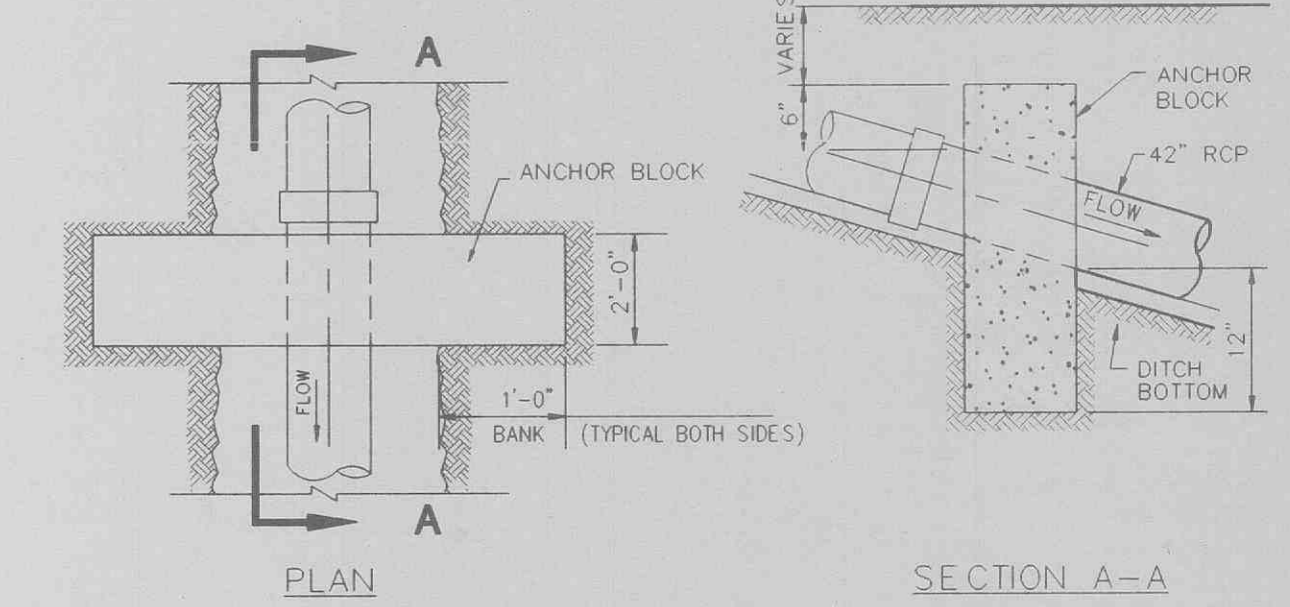
CONCRETE ANCHOR BLOCK N.T.S.
