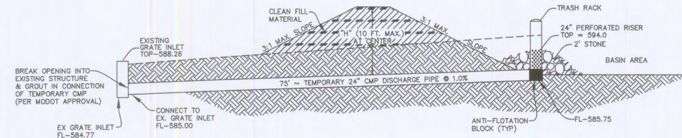
TEMPORARY SEDIMENT BASIN C N.T.S.
