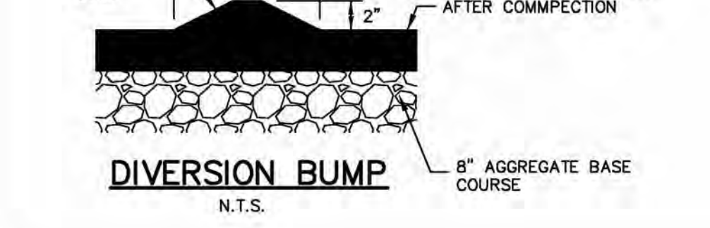
DIVERSION BUMP N.T.S.
