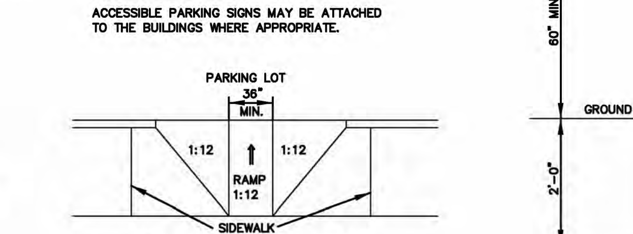
CURB RAMP DETAIL N.T.S.
