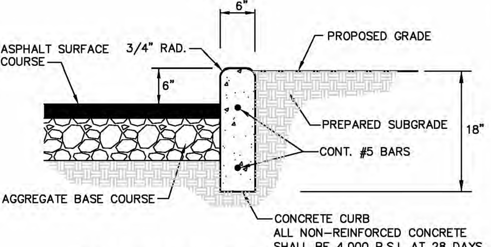
6" VERTICAL CONCRETE CURB N.T.S.
