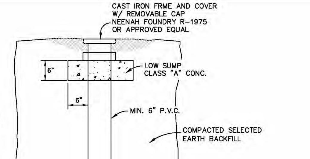
SAMPLE TEE N.T.S.
