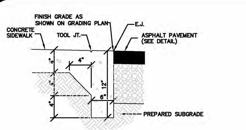
FLUSH CURB DETAIL N.T.S.
