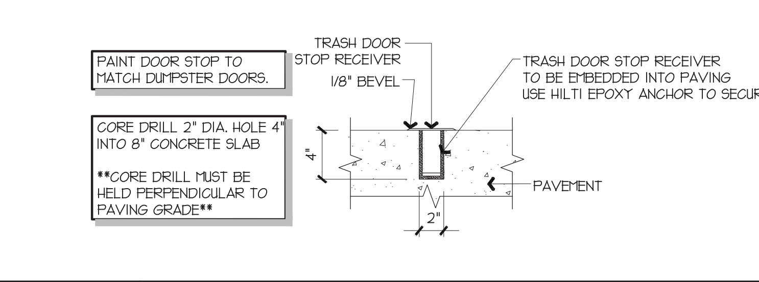
J5 DOOR HOLD OPEN DETAIL
