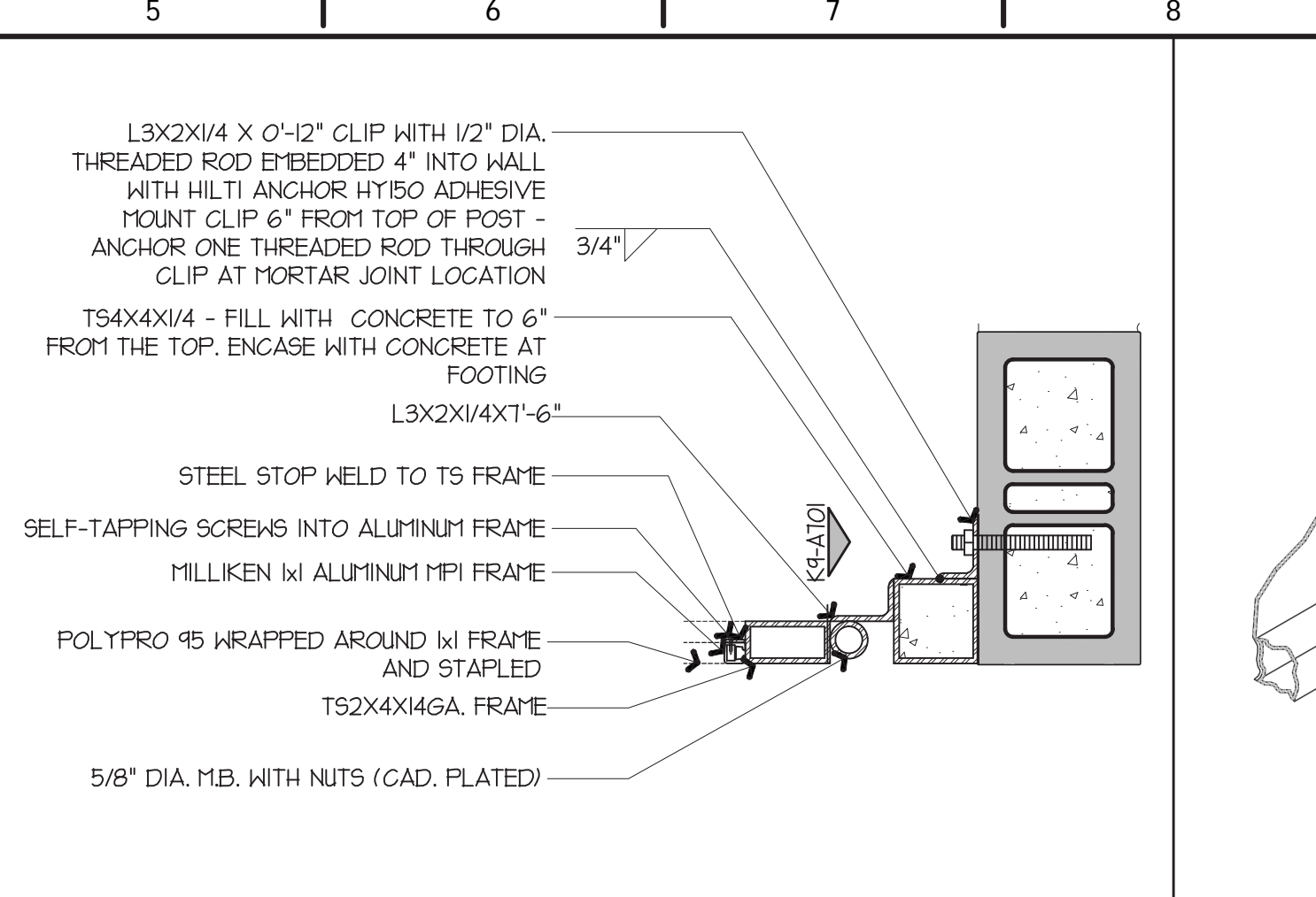
M5 GATE JAMB
