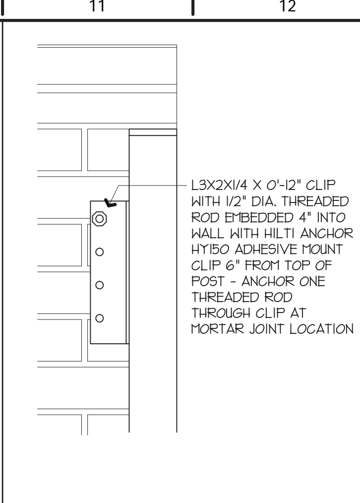
M11 ELEVATION
