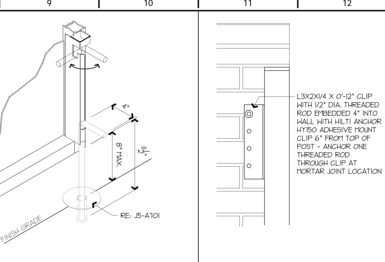
M9 DOOR HOLD OPEN DETAIL
