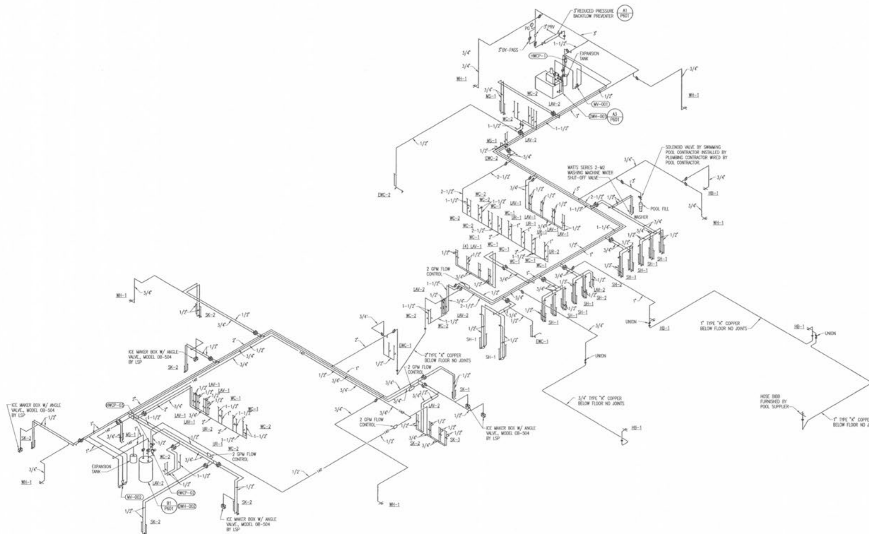
A1 WATER RISER ISOMETRIC SCALE: NONE
