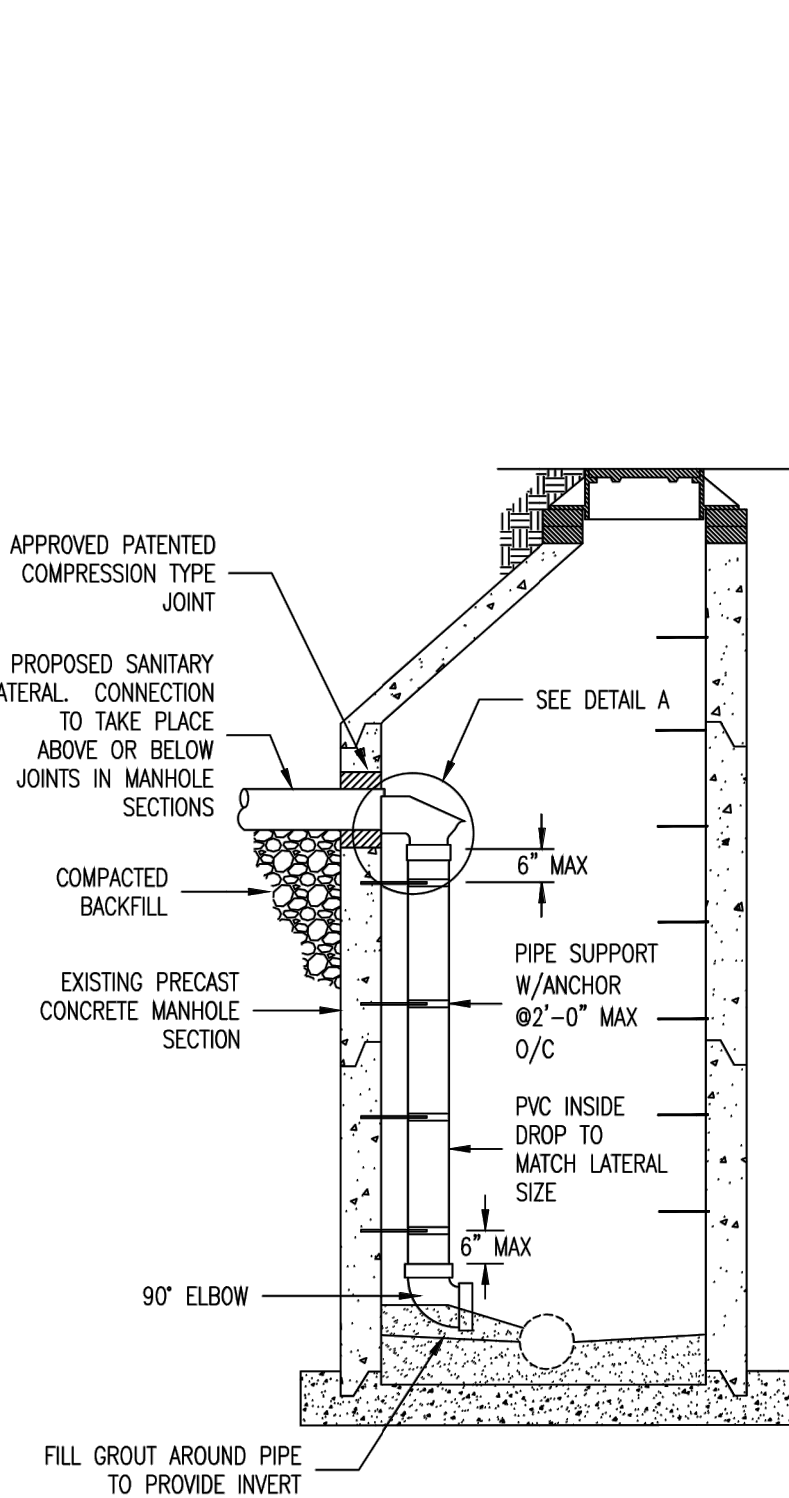
SECTION A-A
