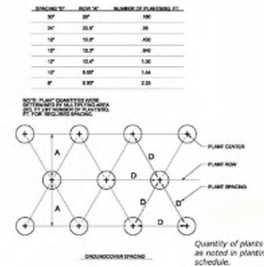
Spacing Diagram N.T.S.
