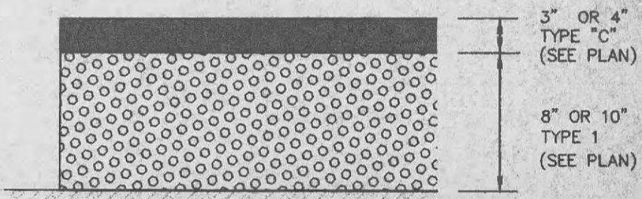
ASPHALT PAVEMENT DETAIL (n.t.s.)
