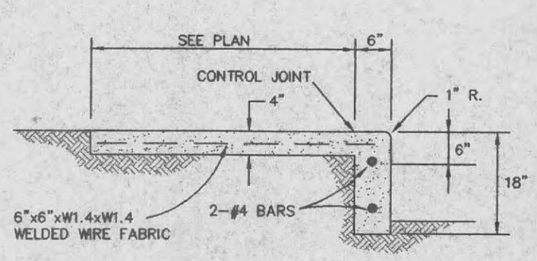
INTEGRAL CONCRETE SIDEWALK & CURB (n.t.s.)
