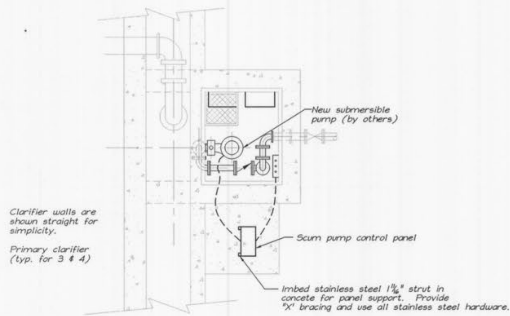
SCUM PIT 3 & 4 - PLAN SCALE: 3/8" = 1'-0"
