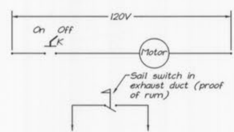
EXHAUST FAN CONTROL No Scale
