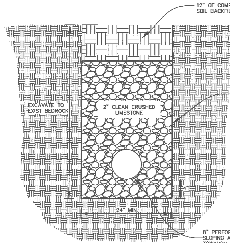
FRENCH DRAIN DETAIL N.T.S.
