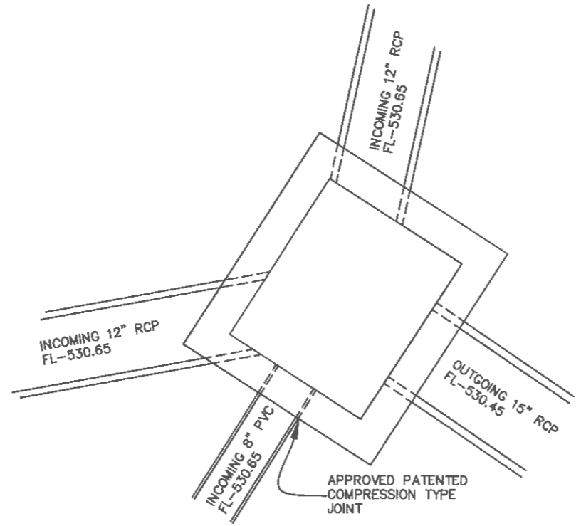
AREA INLET 13 N.T.S.
